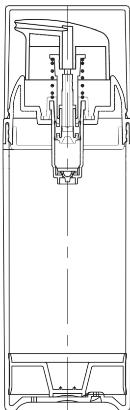
SECCION A-A ESCALA 1:1
