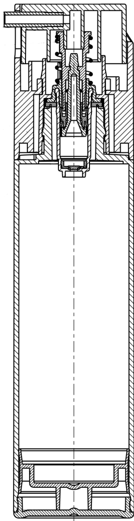
SECCION A-A ESCALA 1:1
