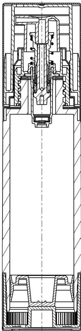
SECCION A-A ESCALA 1:1
